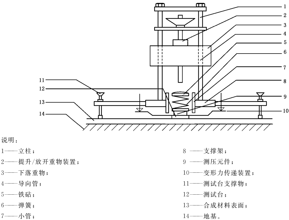
图 E.1 垂直变形测试仪
